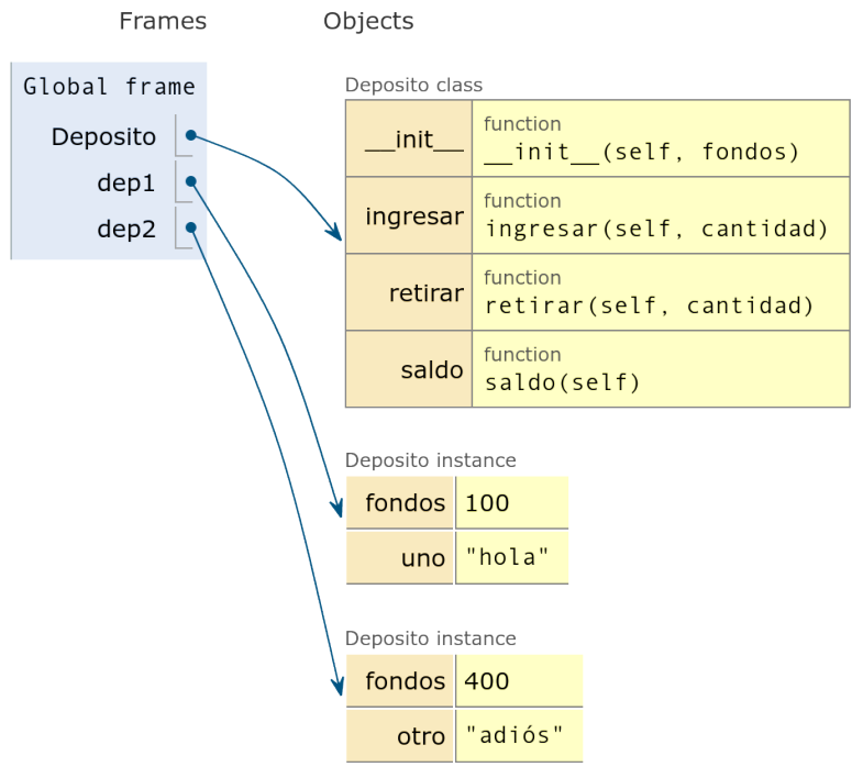
La clase Deposito y los objetos dep1 y dep2 con distintos atributos
